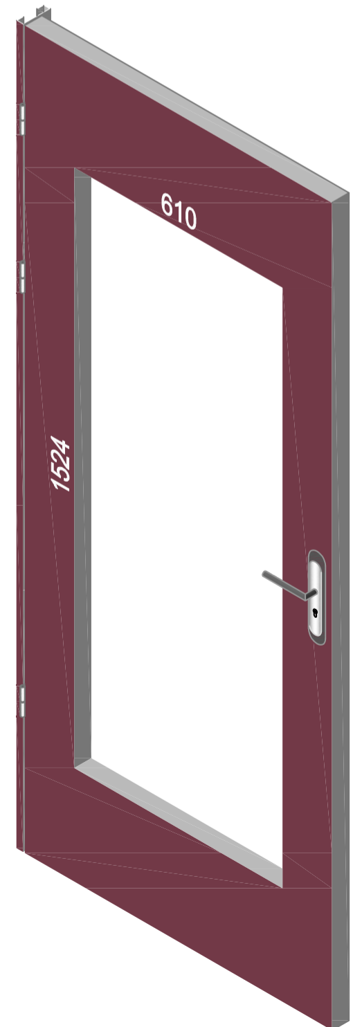
Door Cutout
